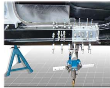
Magnetisches Haltesystem Tragkraft 2 x 35 kg
