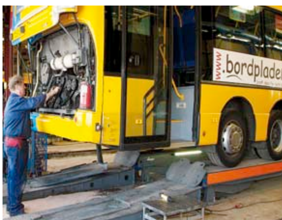
Ergonomisches Arbeiten und optimale Zugänglichkeit bei Reparaturen am Heckmotor.
